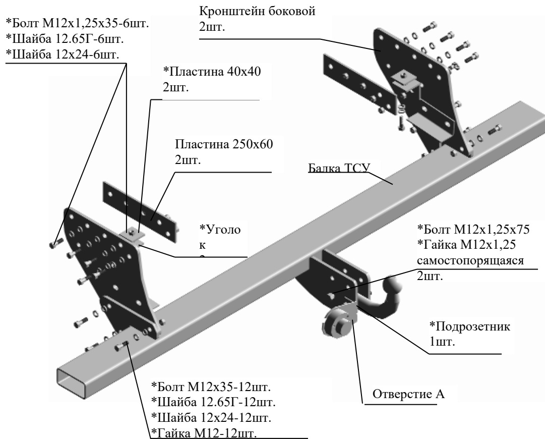
Рис.1 Тягово-цепное устройство 7110.
